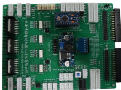
图 3 控制板实物图
